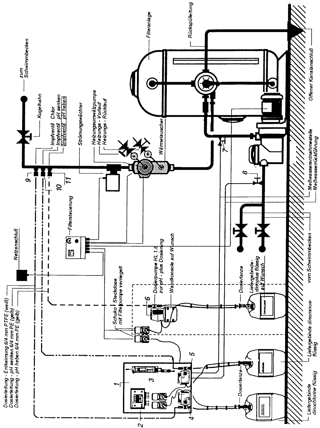
Verrohrungs und Anschlußschema Poolcontrol "Profi" Komplett - Anlage ohne Maßstab
